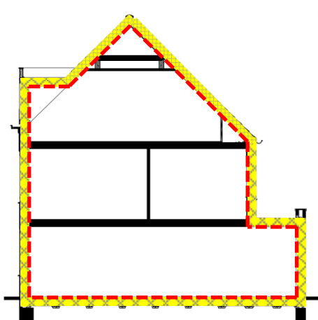
Figuur 2a: Te meten zone valt binnen de thermische schil (= luchtdichte schil); ook de vliering ligt binnen de thermische schil; vliedaken/knieschotten behoren tijdens de meting gesloten te zijn – zie hiervoor paragraaf 5.1.5.
