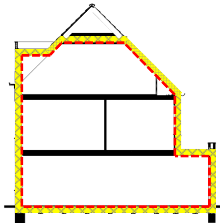
Figuur 2b: Te meten zone valt binnen de thermische schil (= luchtdichte schil); de vliering ligt buiten de thermische schil; vliedaken/knieschotten behoren tijdens de meting gesloten te zijn – zie hiervoor paragraaf 5.1.5.
